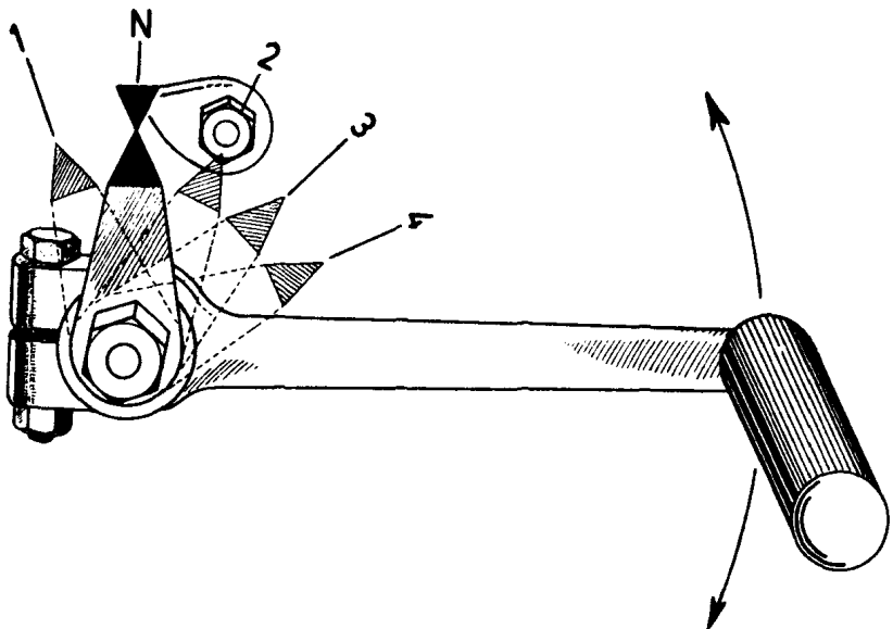
Afb. 5. Het versnellingspedaal
