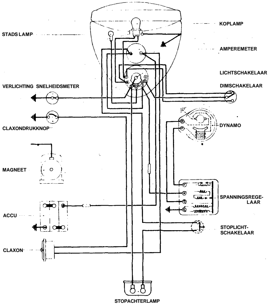
Afb. 11 Het bedradingschema (1949-1951 model)
